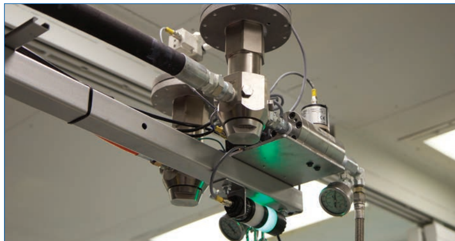
Die grüne Leuchte am System bedeutet, dass die Materialien im korrekten Mischverhältnis dosiert werden.
